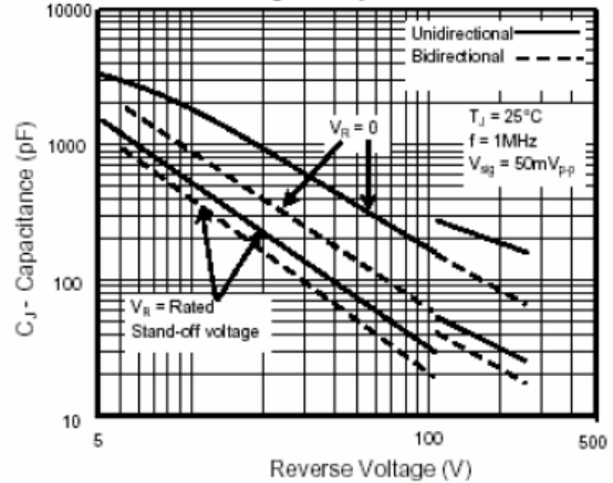
Fig. 6 - Capacitance
